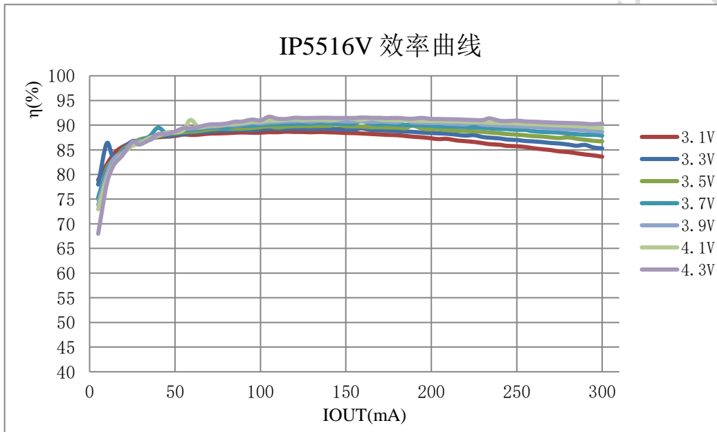
图 4 IP5516V 升压效率图
