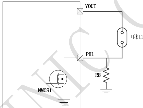
图 10 IP5516V 耳机待机状态的电阻调节原理图
