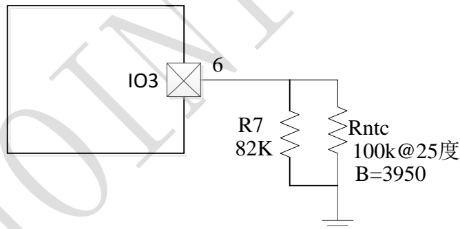
图 9 NTC 电路图
