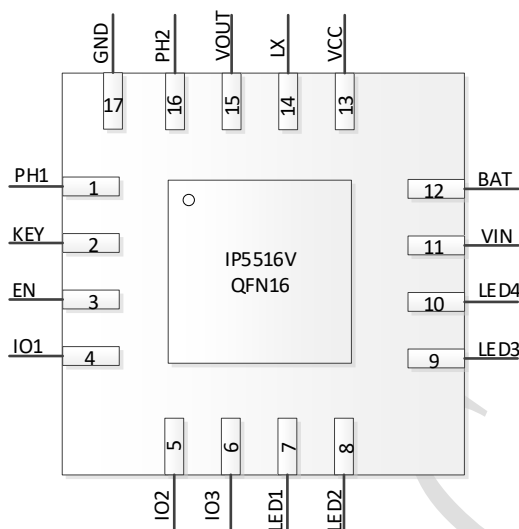
图 2 IP5516V 引脚图
