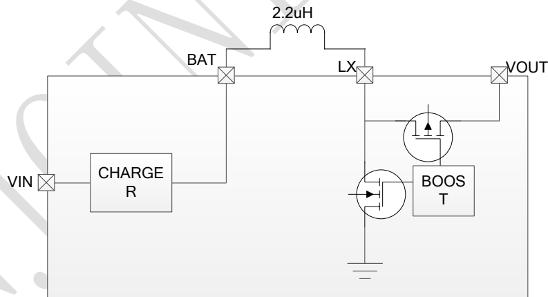
图 7 IP5516V 路径管理示意图
