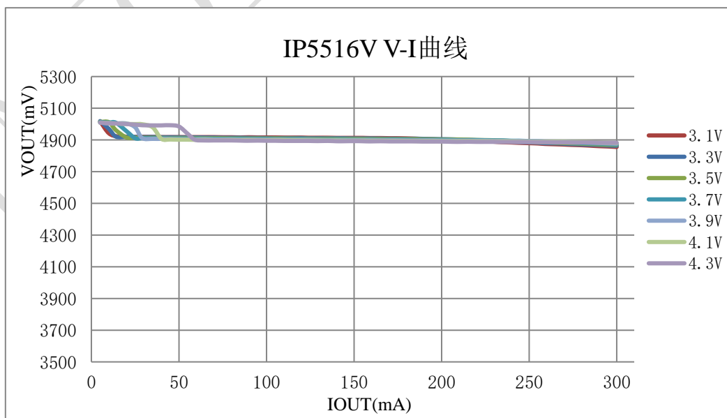
图 5 IP5516V V-I 曲线图
