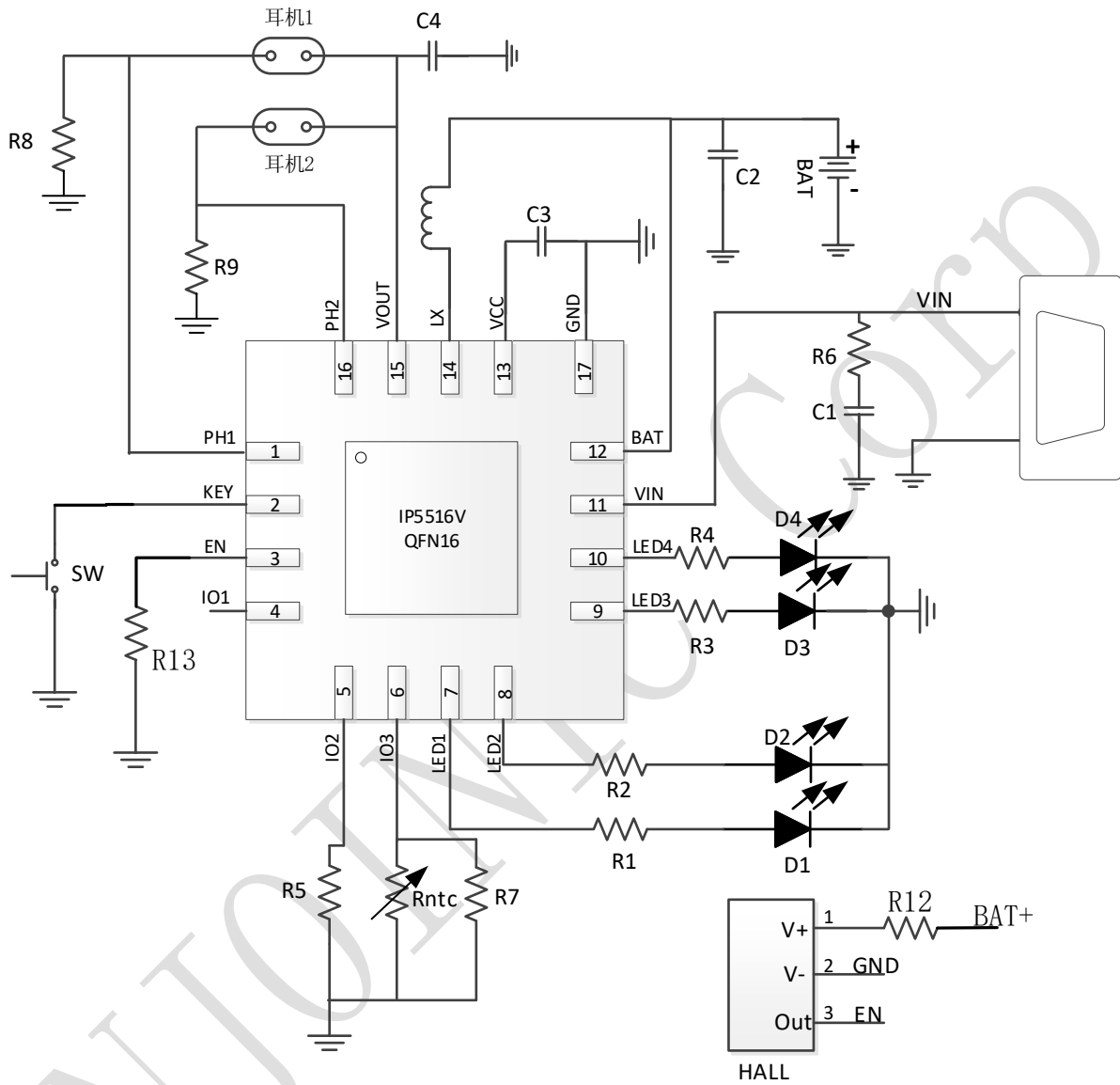
图 1 IP5516V 简化应用原理图
