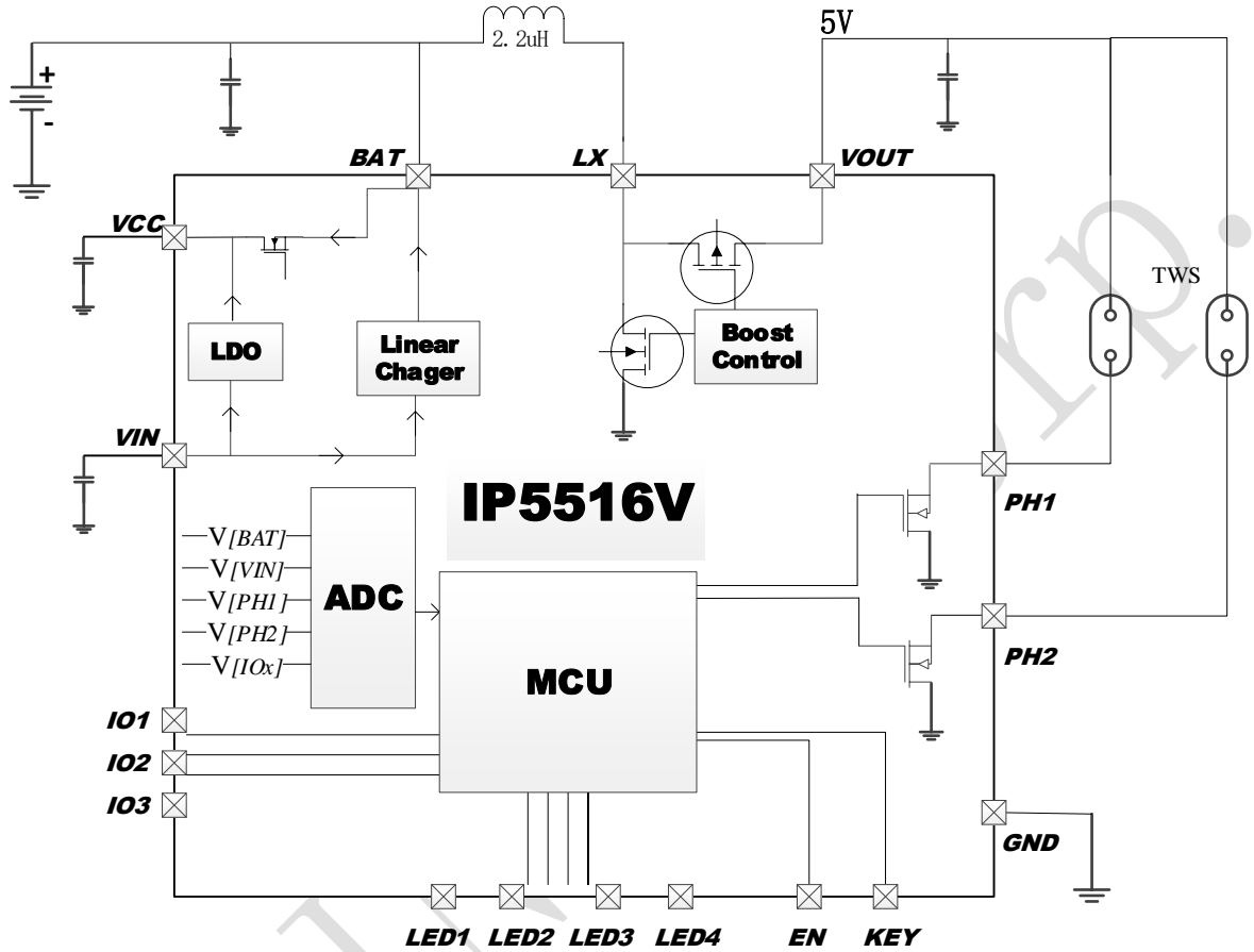
图3 IP5516V 内部系统框图
