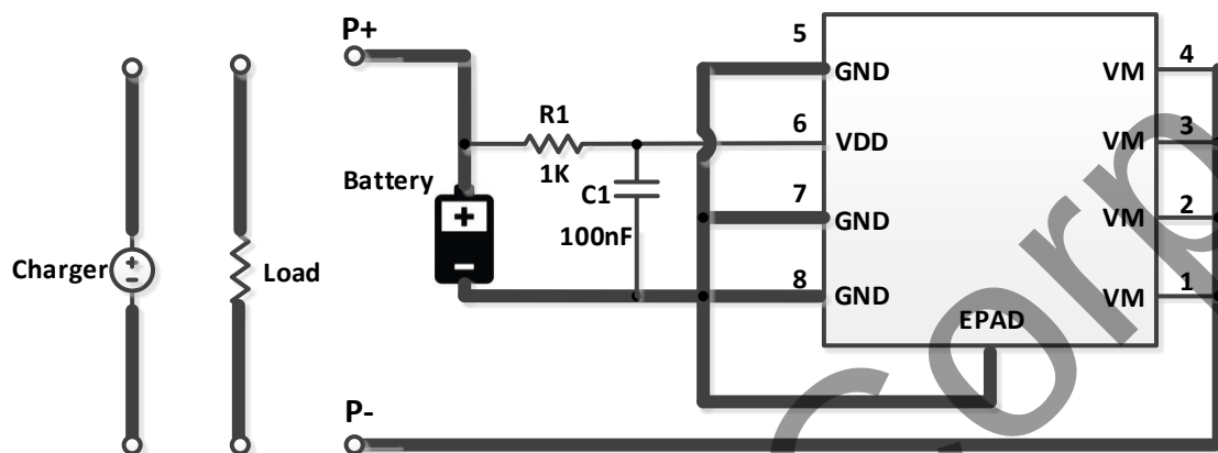
图 8：典型应用图
