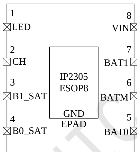
图 2 IP2305 引脚图
