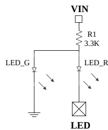
图 5 IP2305_DA_1A 单脚点双灯示意图
