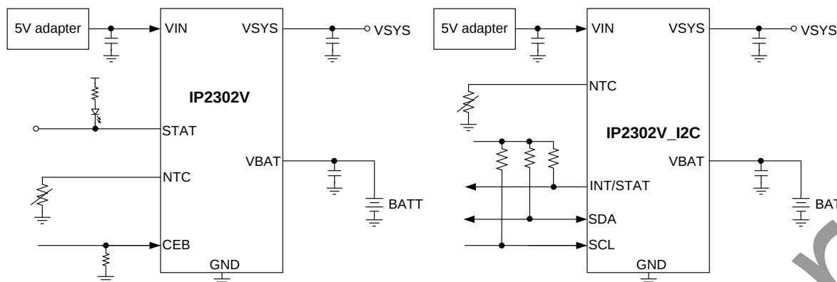
图 1 IP2302V 和 IP2302V_I2C 简化应用原理图
