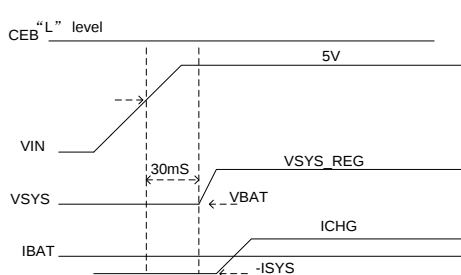
图 5 VIN 启动波形
