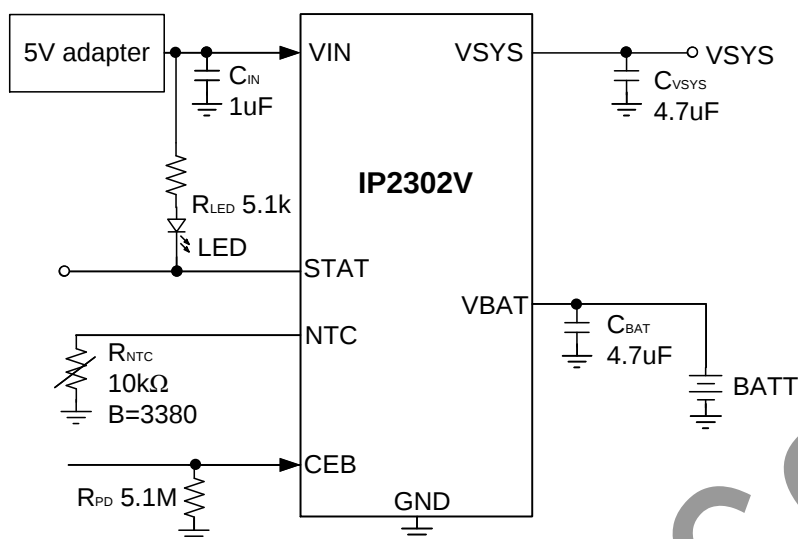
图 11 IP2302V 典型应用原理图
