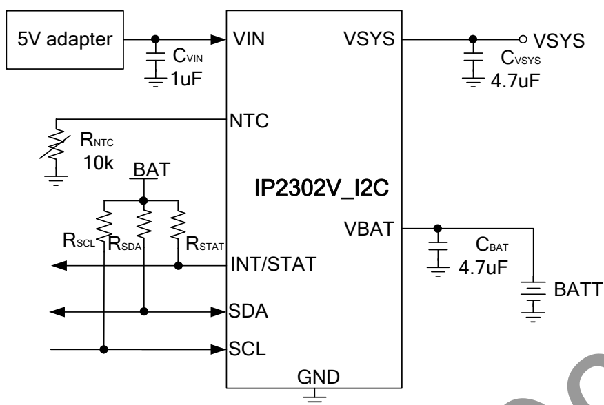
图 12 IP2302V_I2C 典型应用原理图
