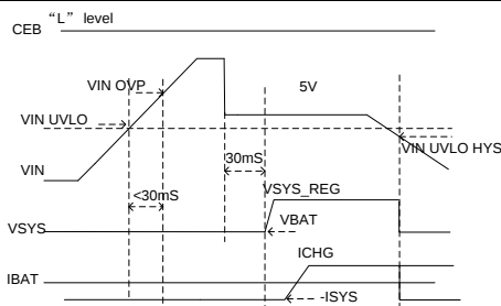
图 6 VIN 过压 OVP 和欠压 UVP 保护
