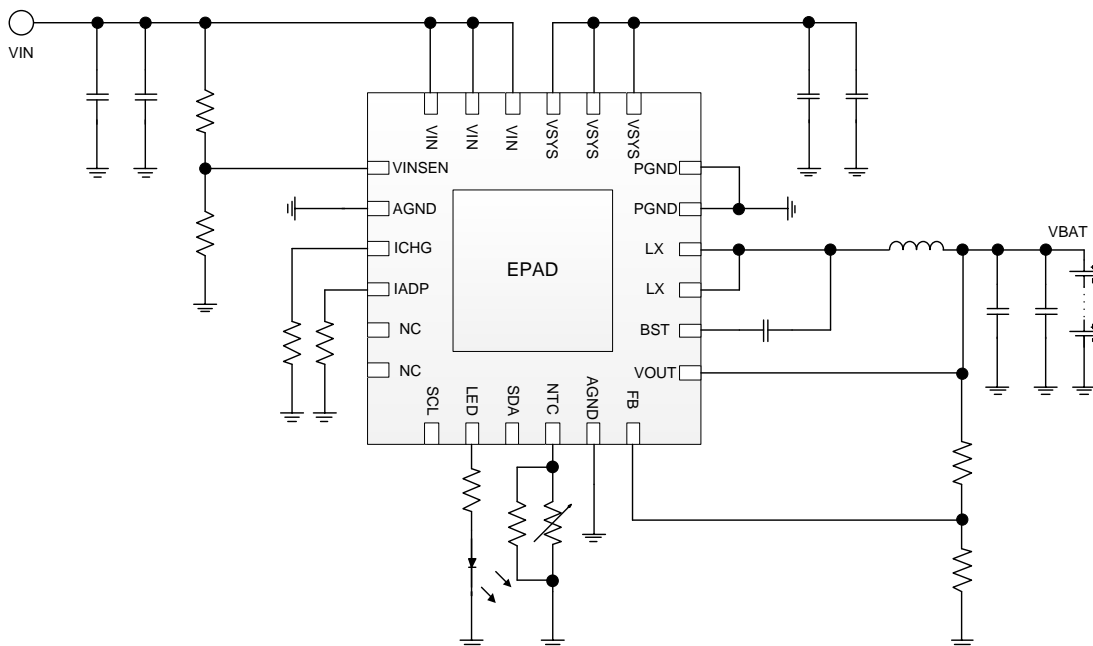
图 1 IP2365 简化应用原理图
