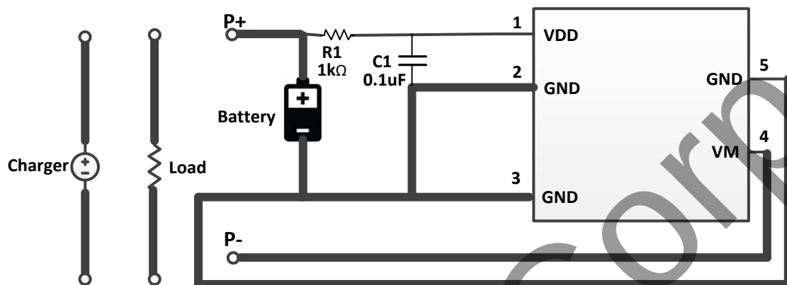
图 8 典型应用图
