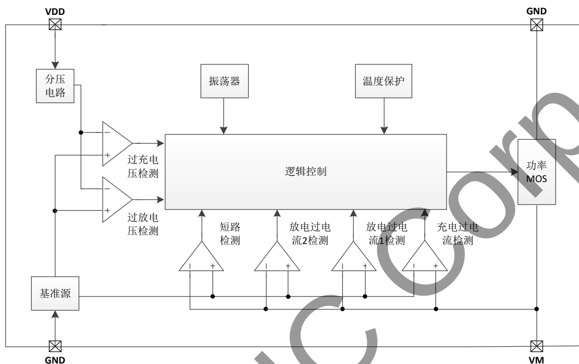
图3 结构框图
