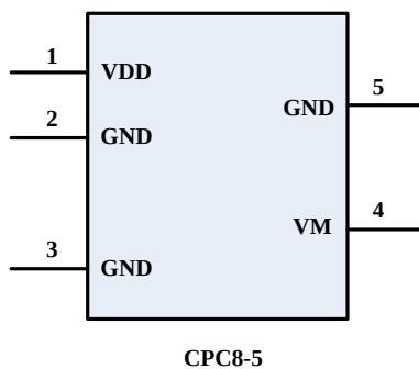
图 2 引脚图
