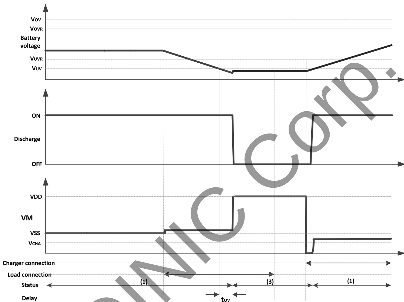
图 6 充电检测
