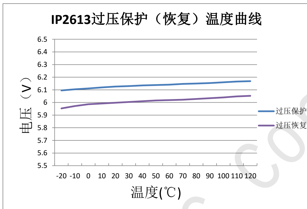
图 9 过压保护（恢复）温度曲线
