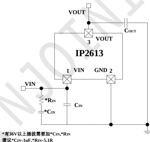
图 1 IP2613 简化应用原理图
