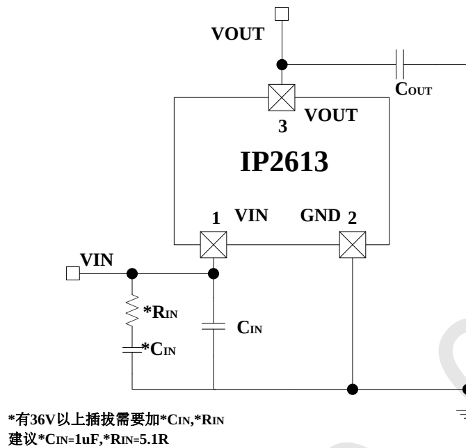
图 10 典型应用原理图
