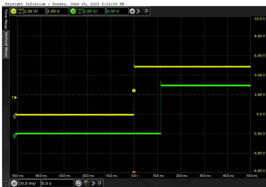
图5 VIN正常上电启动 (VIN=5V)
