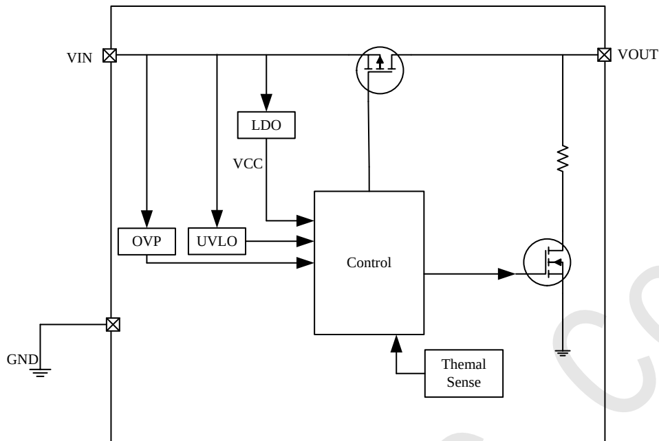
图 3 IP2613 内部系统框图
