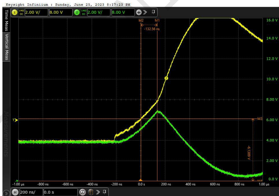
图6 VIN 过压保护 (VIN=5V-15V)
