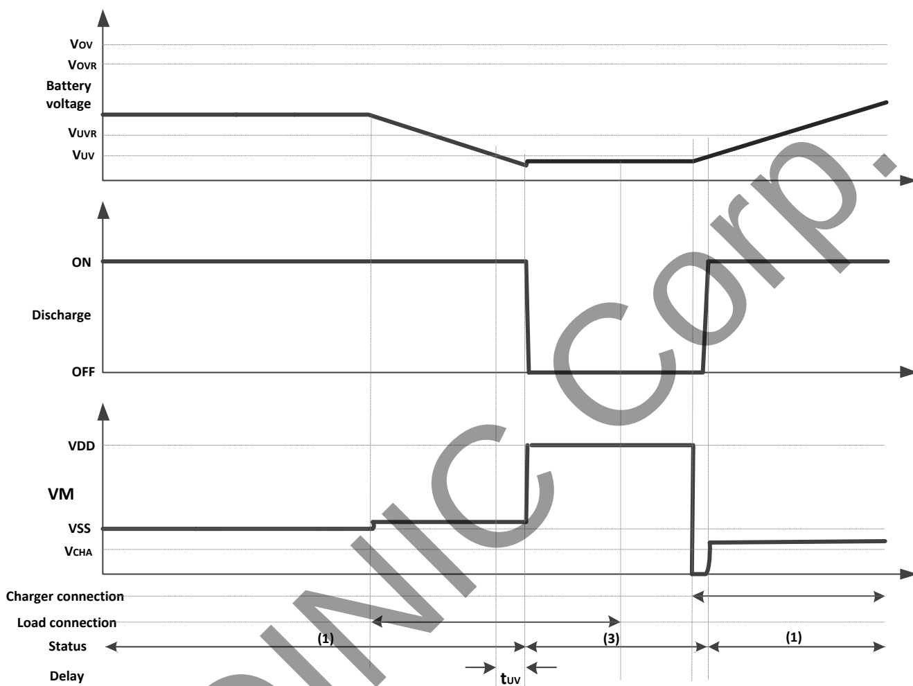
图 6 充电检测
