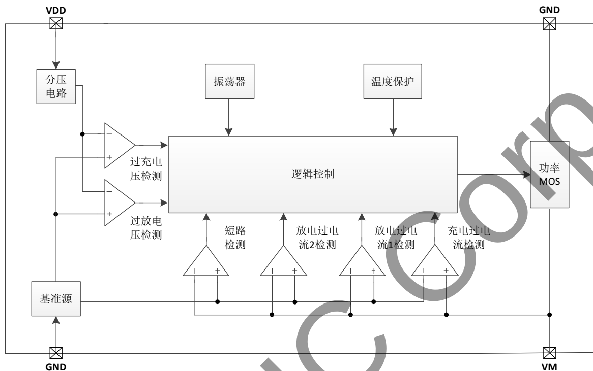
图3 结构框图
