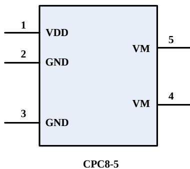
图 2：引脚图
