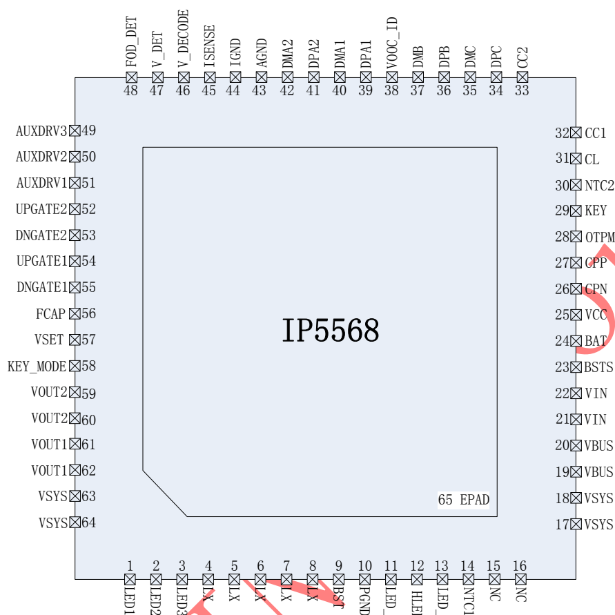
图 2 IP5568 引脚图
